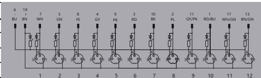
M8-A3-12K3P-M23
